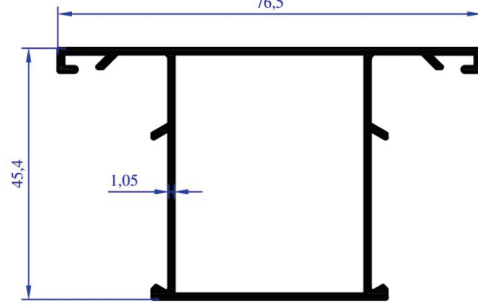
AP 0149 AĞIRLIK 0,569 KG/M DAR ORTA
