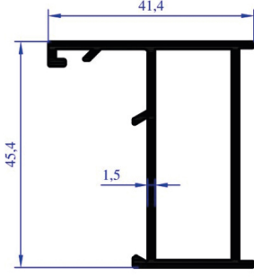
AP 0153 AĞIRLIK 0,656 KG/M DAR KASA
