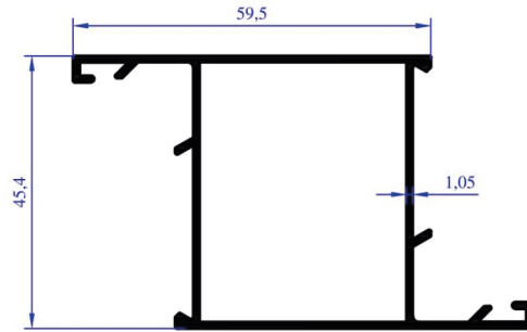
AP 0151 AĞIRLIK 0,569 KG/M DAR KANAT
