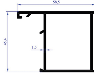
AP 0153 AĞIRLIK 0,656 KG/M DAR KASA
