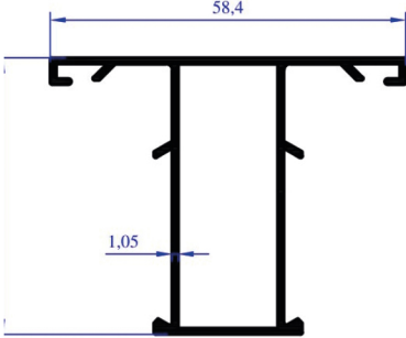
AP 0149 AĞIRLIK 0,569 KG/M DAR ORTA
