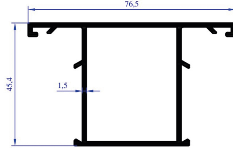
AP 0156 AĞIRLIK 0,921 KG/M GENİŞ ORTA
