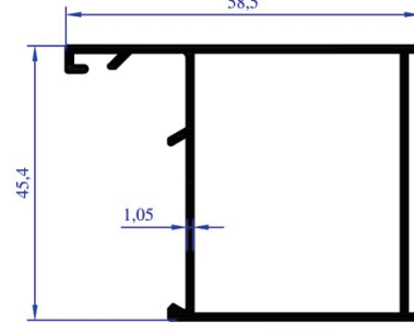
AP 0149 AĞIRLIK 0,577 KG/M GENİŞ KASA
