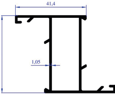
AP 0151 AĞIRLIK 0,569 KG/M DAR KANAT
