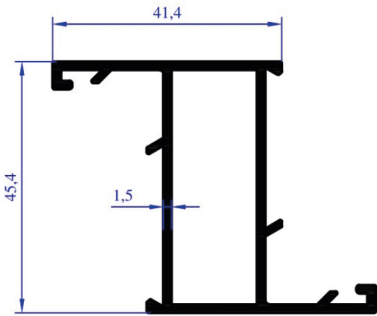
AP 0157 AĞIRLIK 0,775 KG/M DAR KANAT
