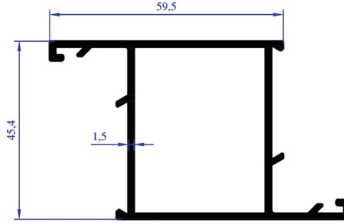
AP 0158 AĞIRLIK 0,921 KG/M GENİŞ KANAT
