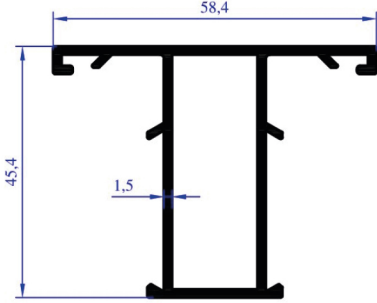
AP 0155 AĞIRLIK 0,775 KG/M DAR ORTA
